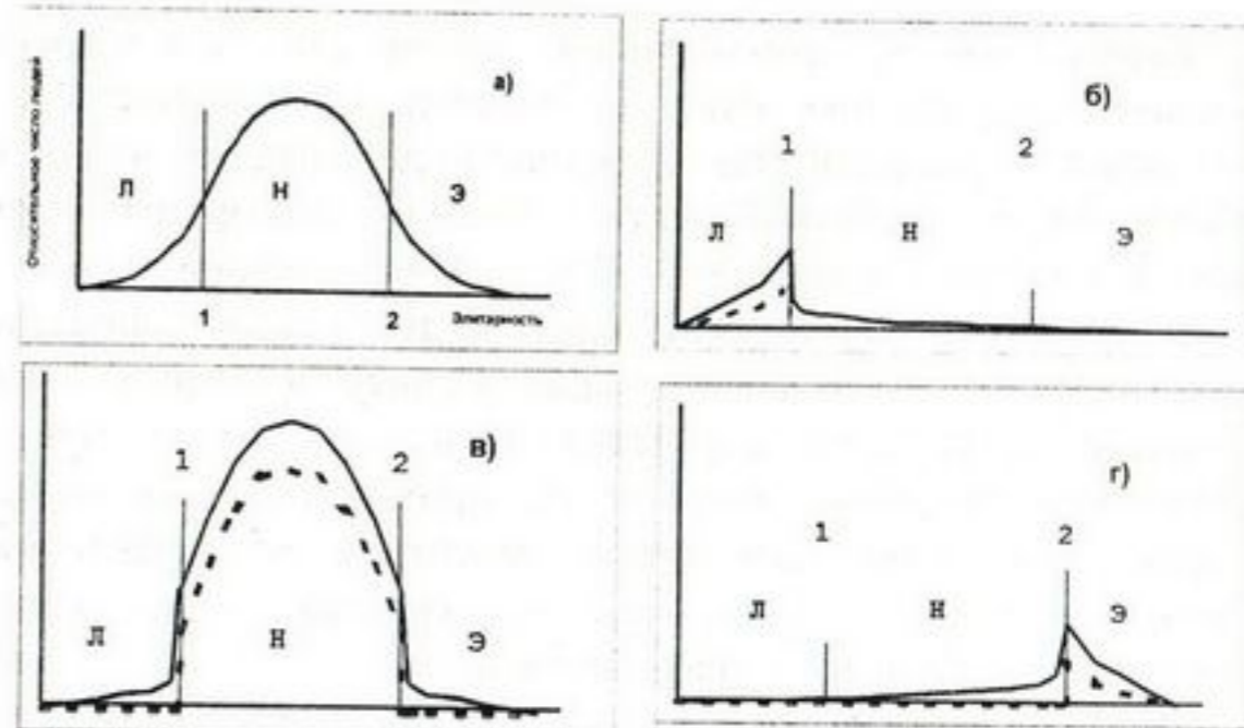
Рис. 4. Влияние закона изменчивости на элитарное распределение потомства в зависимости от элитарности родителей из различных элитарных групп: а) исходная популяция; б) распределение потомства из люмпенов; в) распределение потомства из народа; г) распределение потомства из элиты.
