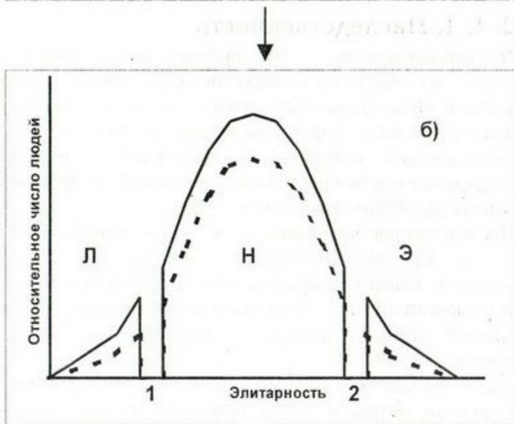
Рис. 3. а) Распределение числа людей в популяции в зависимости от элитарности: Л — люмпены, Н — народ, Э — элита; 1 и 2 — условные границы соответственно между люмпенами и народом, и между народом и элитой.
